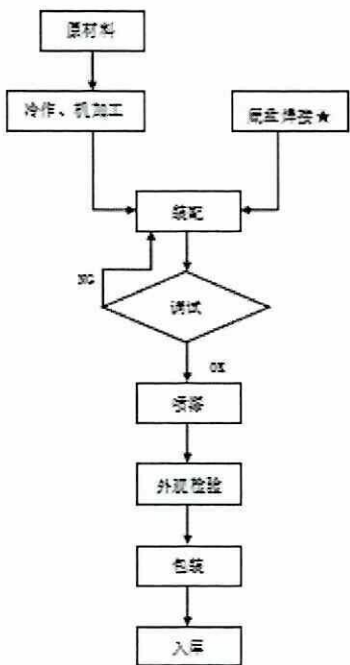
图 3-1-2 主要生产工艺流程图
